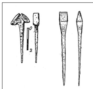
Abbildung 5: Eisnägel. Burg Rickenbach, 13. Jahrhundert (Meyer – Hofmann W., 1972) und 20. Jahrhundert (Schwendimann F., o. Jg.).
